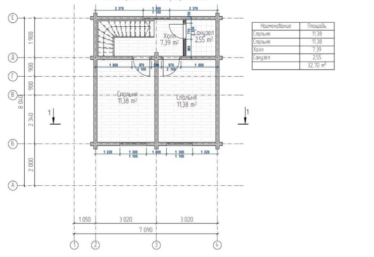
План второго этажа (маркировочный)
