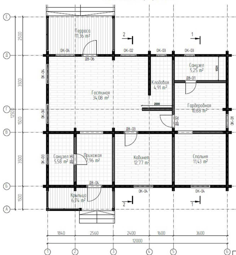
План этажа (маркировочный)
