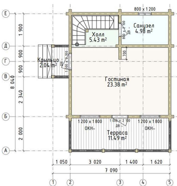
План первого этажа (маркировочный)
